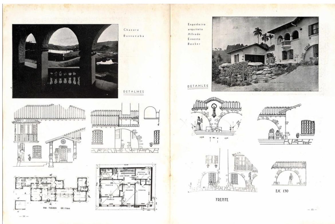
Figura 11: Imagens, plantas e detalhes da Chácara Bussucaba projetada por Alfredo Ernesto Becker.
