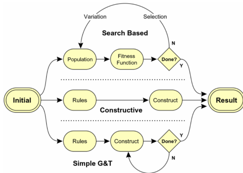
Figura 4.1: Fluxogramas comparativos de diferentes técnicas PCG.
