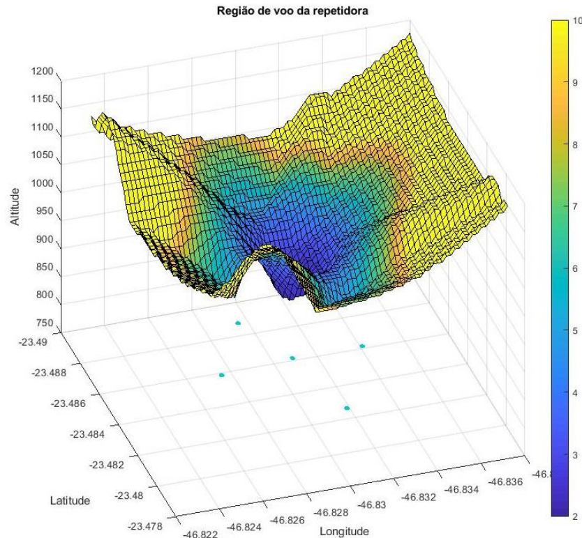
Figura 6 – Gráfico de superfície da região de voo da repetidora
